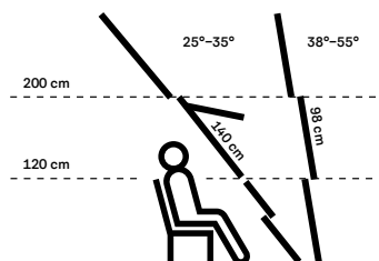
Finestra con apertura a vasistas (con comando dal basso) singola e in combinazione con un elemento sottostante
