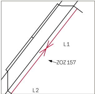
Apertura nel tetto (rivestimento interno) oltre 240 cm
