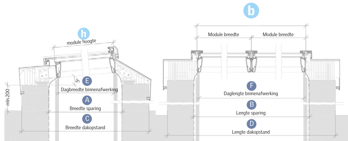
Dwarsdoorsnede-Lessenaarsdak
