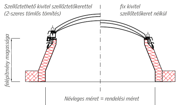
Top 90 felülvilágító kupola ISO-THERM lábazon
