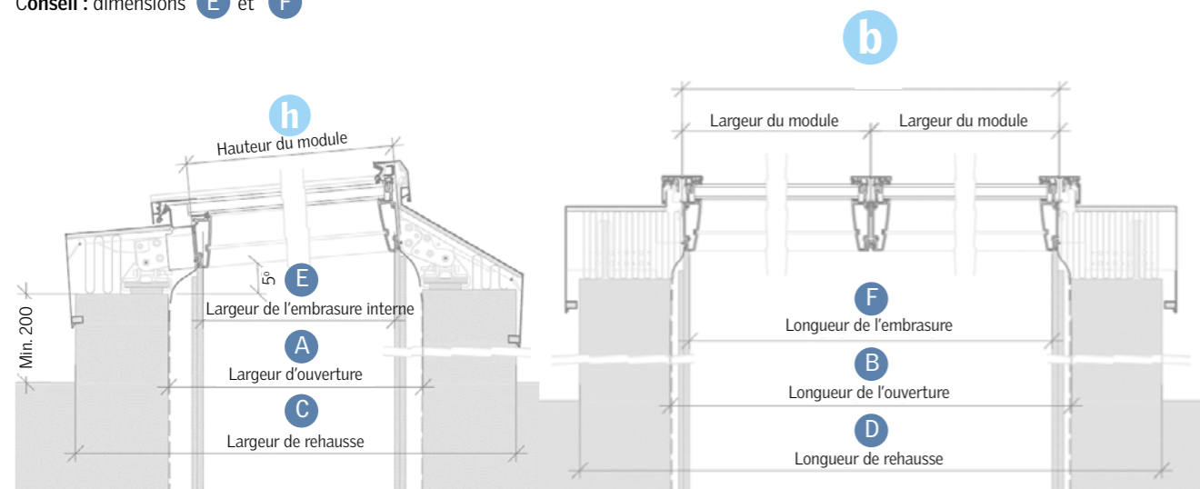
Section transversale - Verrière linéaire
