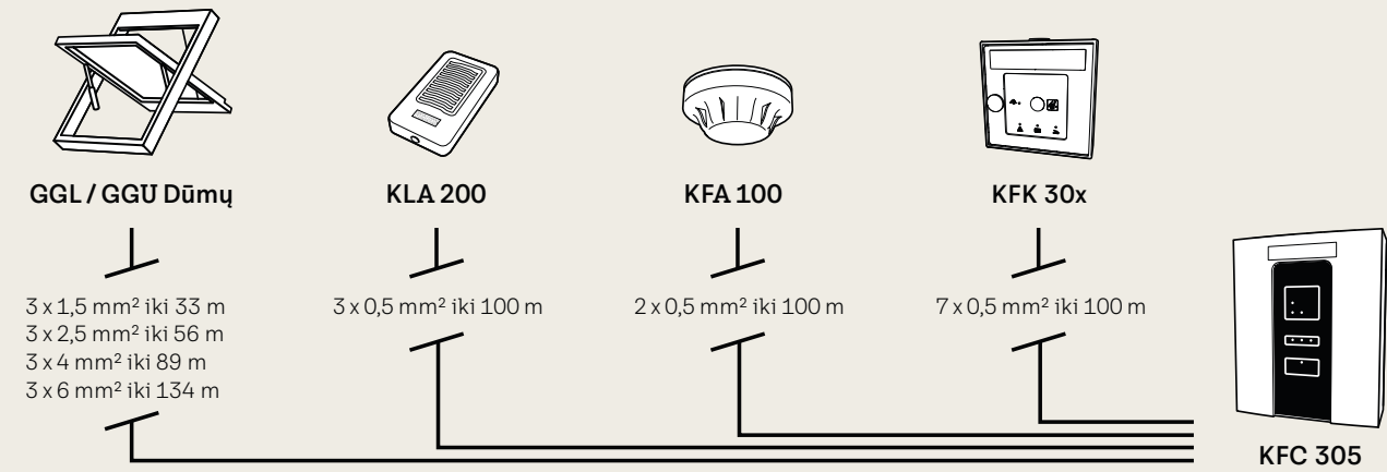
Prijungimo schema šlatiniams stogams
