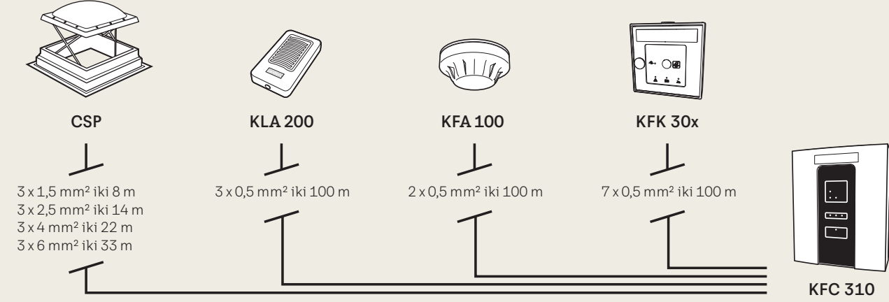
Prijungimo schema plokšties stogams
