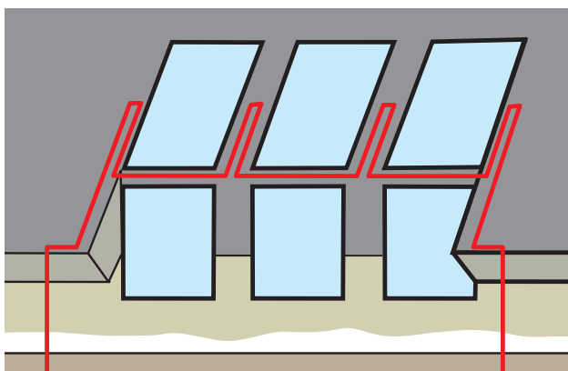
Prinsipp for varmekabler ved innbygging med fasadelementer
