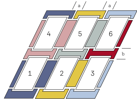
6er-Kassette
