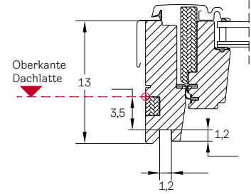
Vertiefter Einbau
