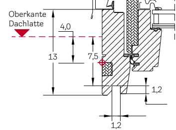
Vertiefter Einbau
