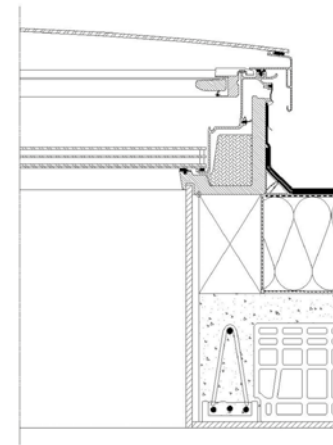
Ventana Salida a Cubierta con Cúpula Vidrio Liso CXU + ISU
