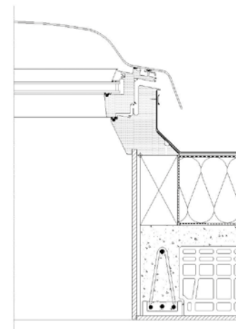
Ventana Salida a Cubierta CXP + ISD
