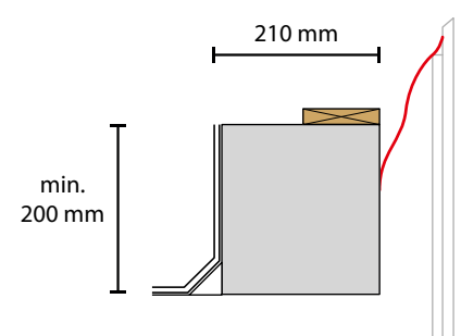
Holz mit Holzleiste
