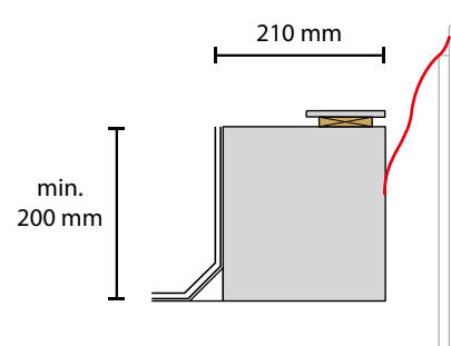
Beton mit Flachstahl
