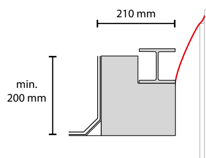
Beton mit Stahlprofil
