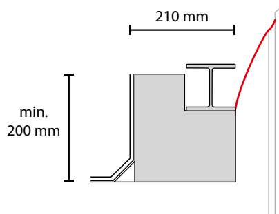
Stahl mit Stahlprofil
