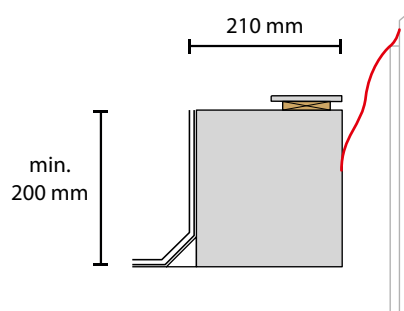
Stahl mit Flachstahl
