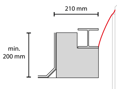
Holz mit Stahlprofil
