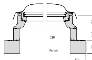
Finestre per tetti piani CSP EFC con telaio di estensione fisso. Con telaio di estensione addizionale in Purenit
