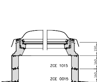
Finestre per tetti piani CVP/CFP con telai di estensione ZCE 0015 e ZCE 1015 versione set ZCE S000
