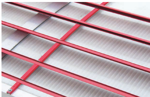
VARIO-PROTECT 120 VWS na łukowym paśmie świetlnym
