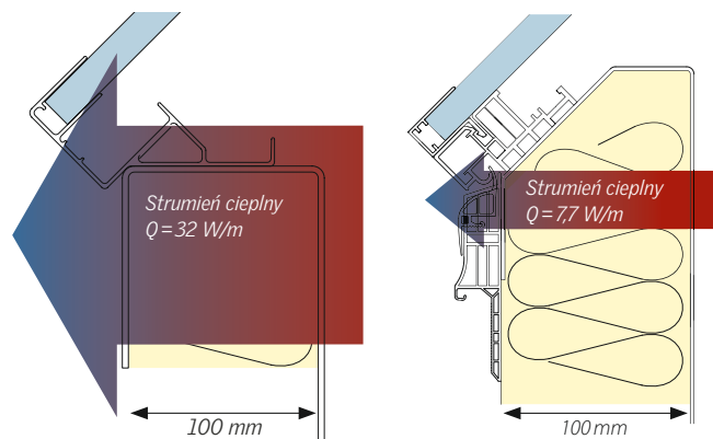
Strumień ciepły w tradycyjnych konstrukcjach Strumień ciepły VARIO-THERM-S
