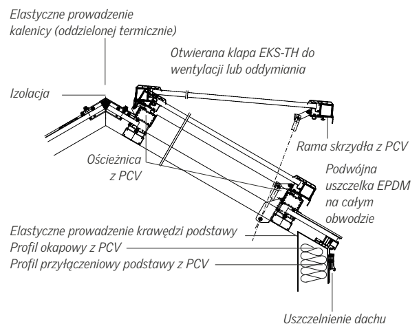
Przekrój przez dwuspadowe pasmo świetlne VARIO-THERM-S z klapą EKS
