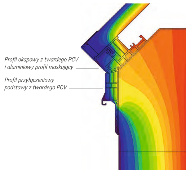
Strumień ciepły w tradycyjnych konstrukcjach Strumień ciepły VARIO-THERM-S
