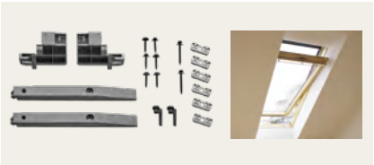
ZOZ 238 Montagekit für Elektro- und Solar-Markisetten Für Montage auf VELUX Dachfenster GGU/GGL in den Größen 102–810
