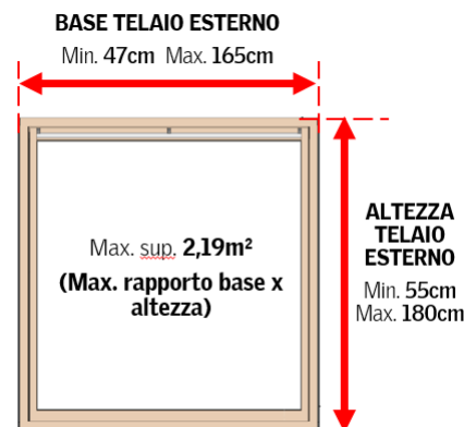
Fig.2 Regole finestre fuori misura
