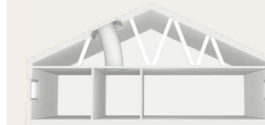
Šviesos tunelis lanksčiu vamzdžiu šlaitiniam stogui
